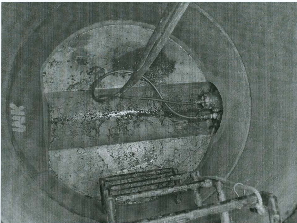
Fotografia č. 3 – SO Jalovec – tlakovanie úseku
