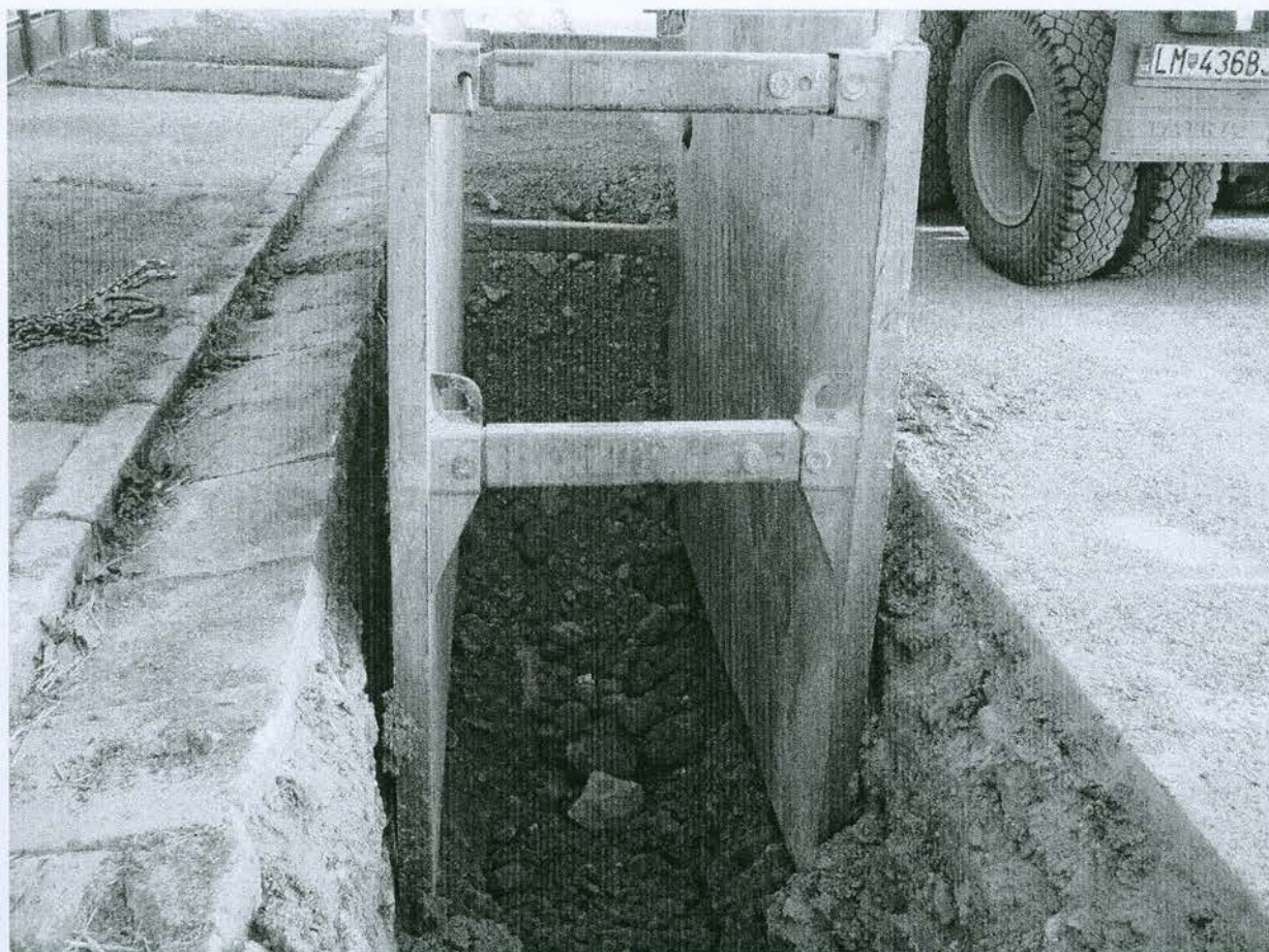
Fotografia č. 7 – SO Závažná Poruba – Dosypávanie výkopu zeminou
