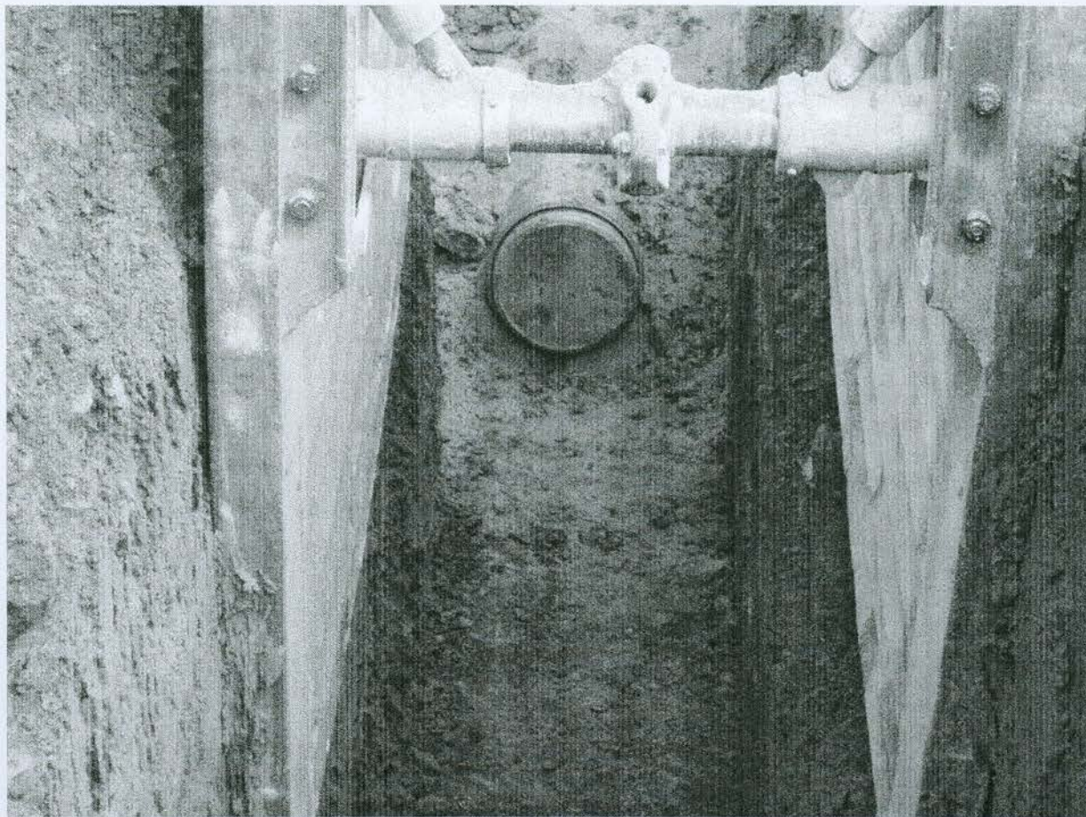
Fotografia č. 5 – SO L. Mikuláš Stošice – Uzavretie DN 300 zátkou
